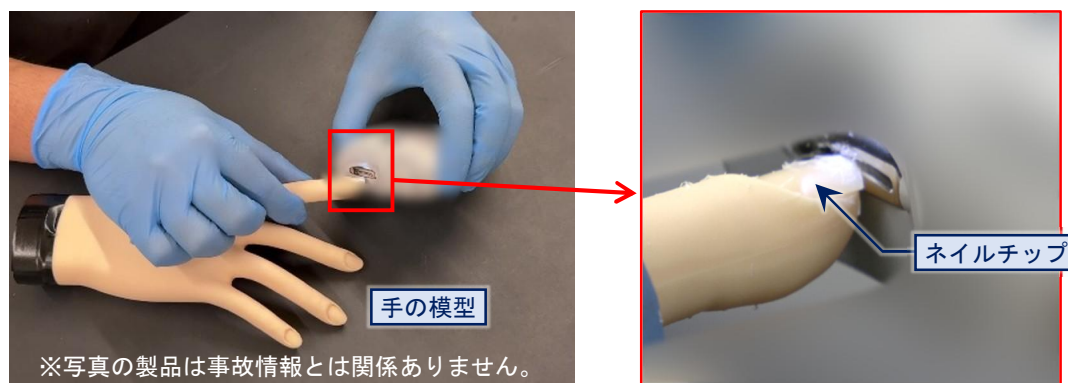
図 7 爪削りテストの様子
