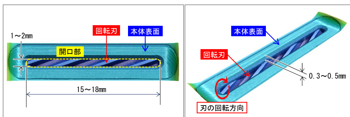
図 6 開口部及び回転刃の 3D モデル
