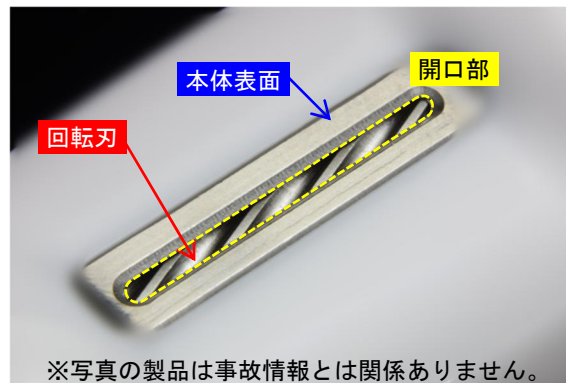
図3 開口部及び回転刃の例
