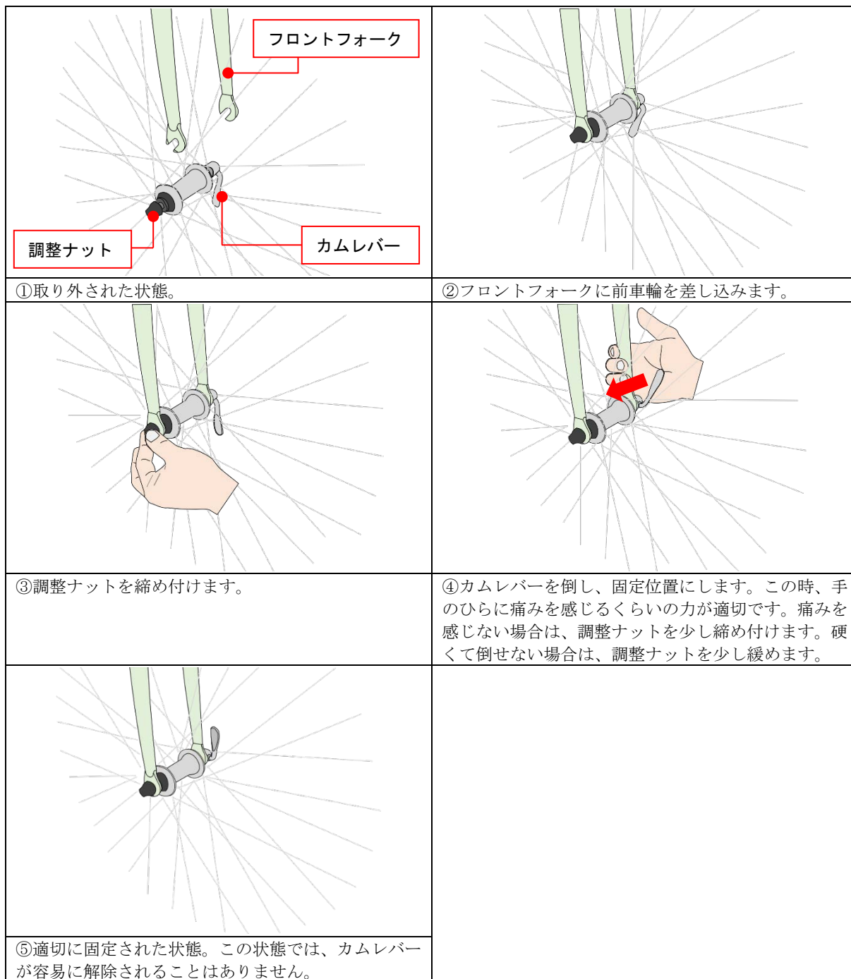
図2. クイックリリースハブの正しい固定手順
