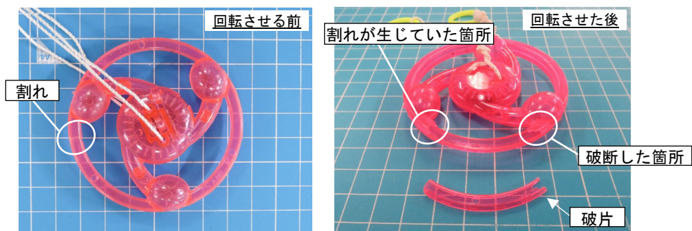
写真4. 回転させたことで破断した同型品の様子
