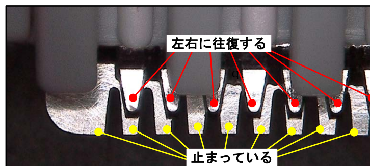
写真1. 刈刃の外観
