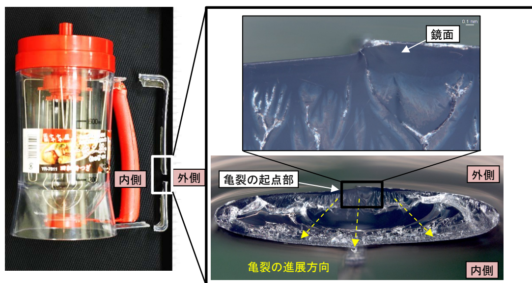
写真2. 破損部の破面
