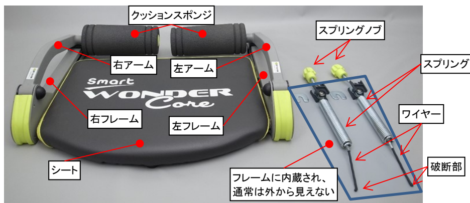
写真1. 調査した当該品の外観と各部名称
