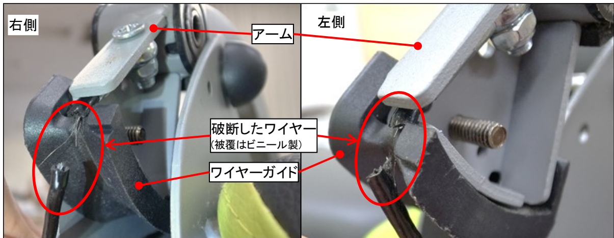
写真2. ワイヤー破断部
