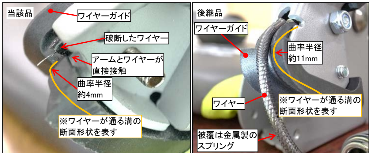
写真3. 調査した当該品と該当する商品の後継品のワイヤーガイド
