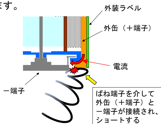
（図3）アルカリ乾電池のショート
