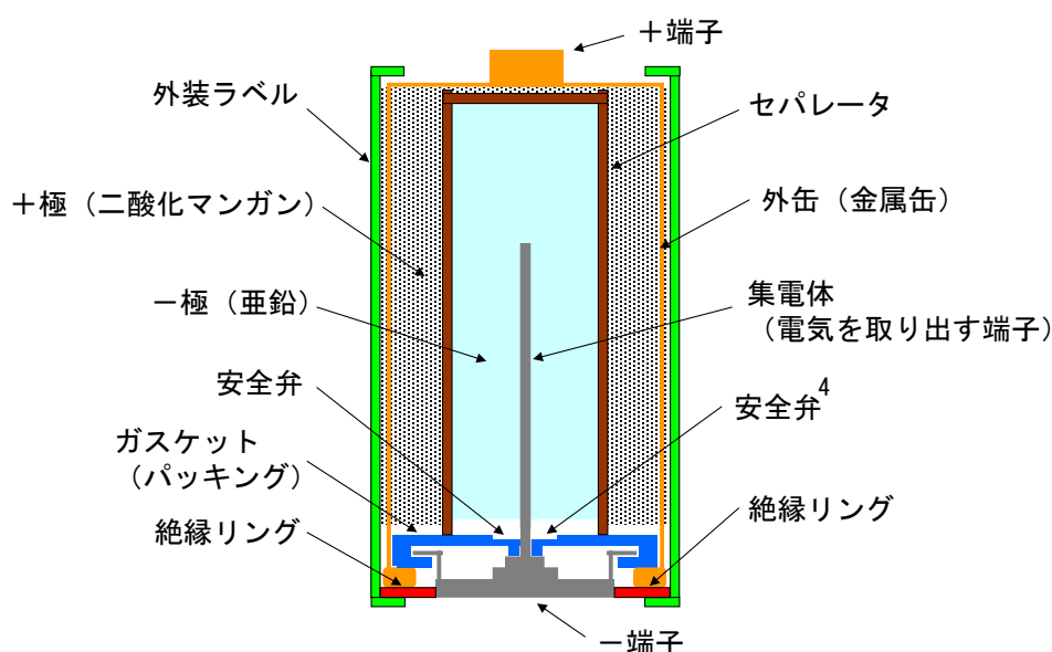
(図2) アルカリ乾電池の内部構造
