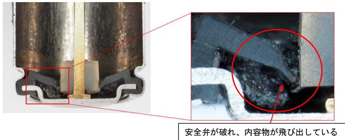
(写真5) アルカリ乾電池内部の安全弁の様子
