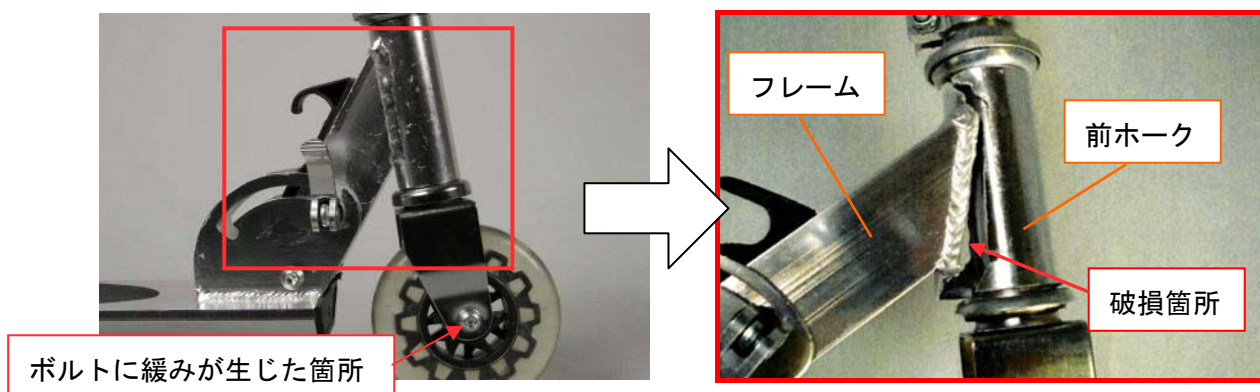
写真 2. 破損、ボルトの緩みが見られた箇所（一例）
