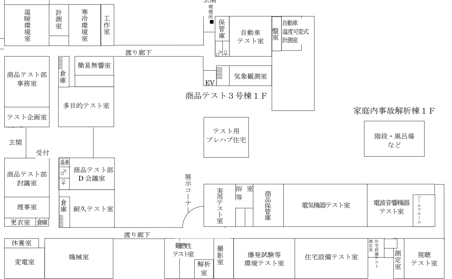
商品テスト 1号棟 2号棟 3号棟 1階図
